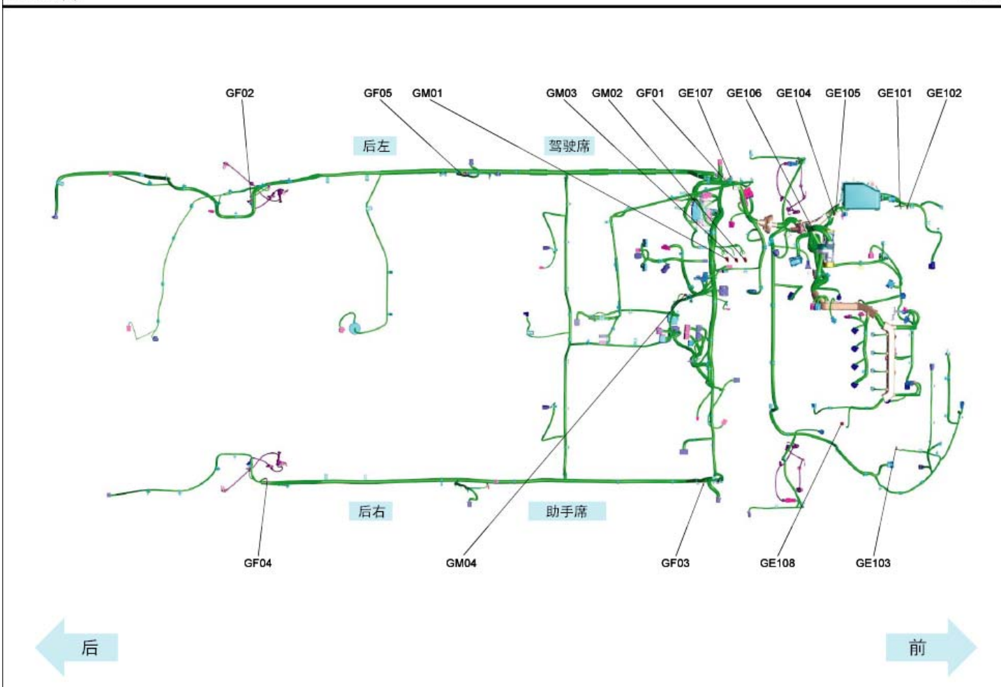
搭铁点(1)
